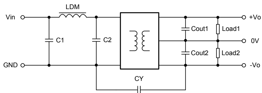
图 2 EMC 推荐电路图
