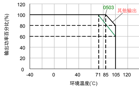
环境温度降额曲线图
