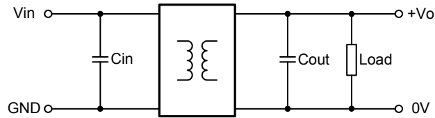
图 1 应用电路图
